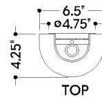
TOP
